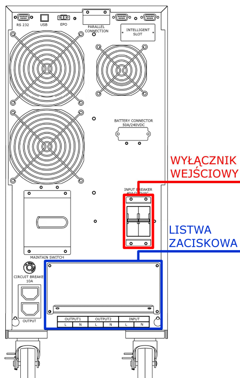
Panel tylny UPS
