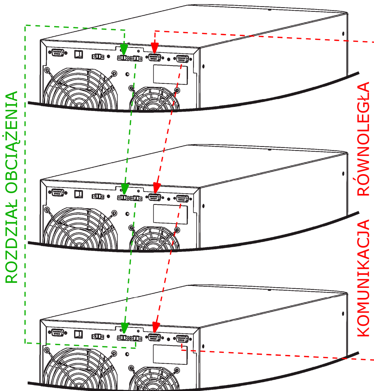
Schemat połączenia komunikacji
