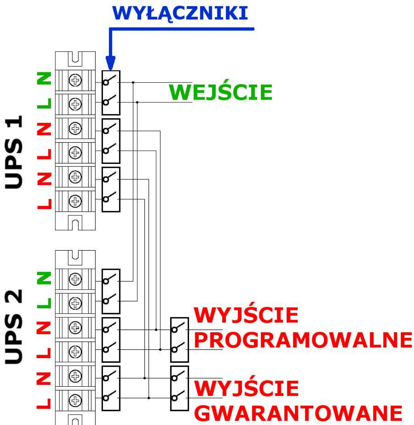
Schemat połączenia wejść i wyjść
