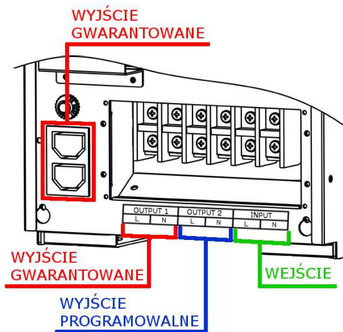
Listwa zaciskowa
