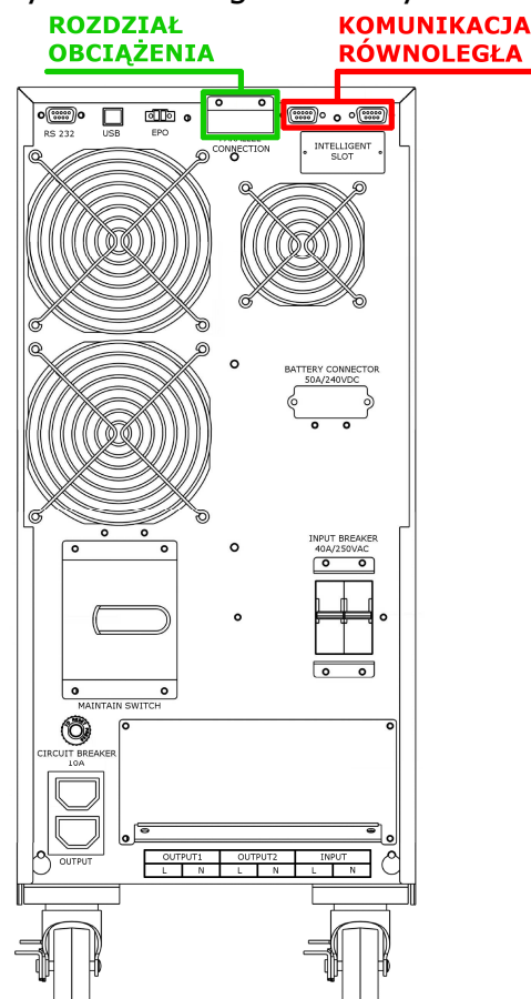
Panel tylny UPS
