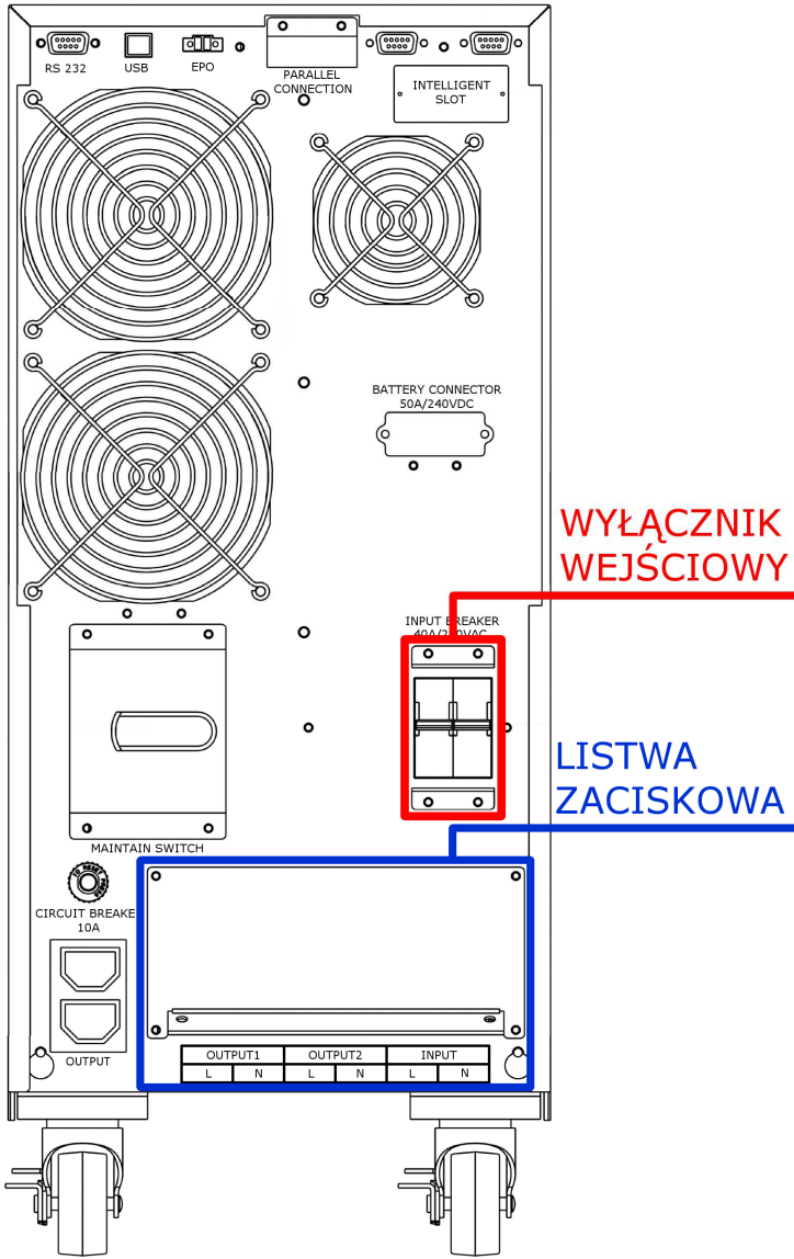
Tylny panel UPS
