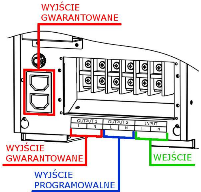
Listwa zaciskowa
